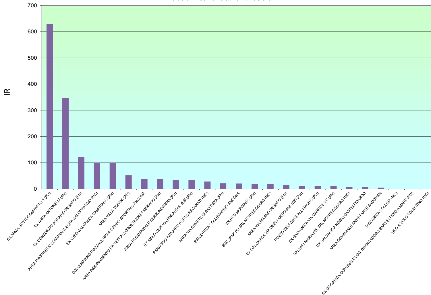
Indice di Rischio Relativo Atmosfera
