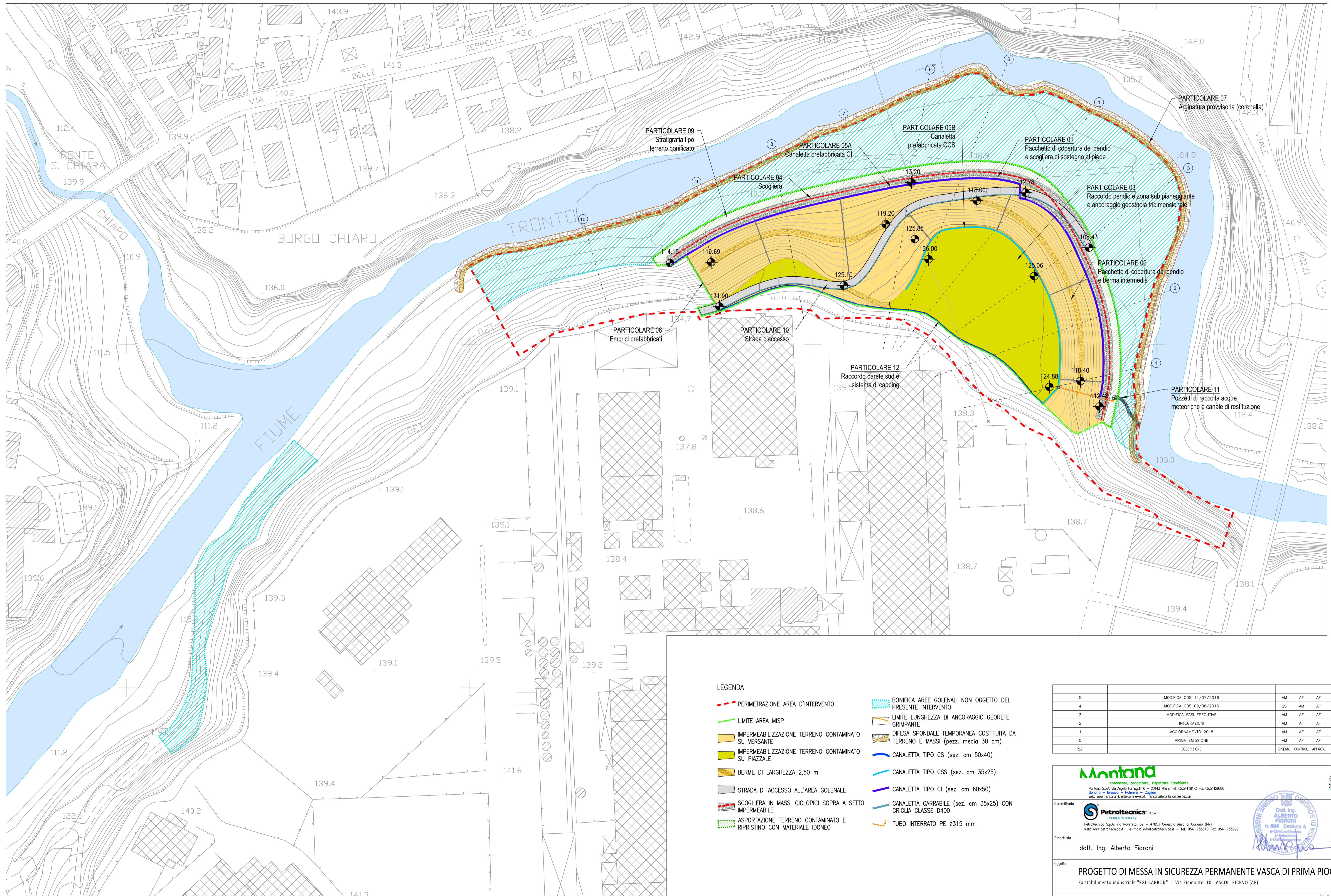
PLANIMETRIA GENERALE STATO DI PROGETTO
