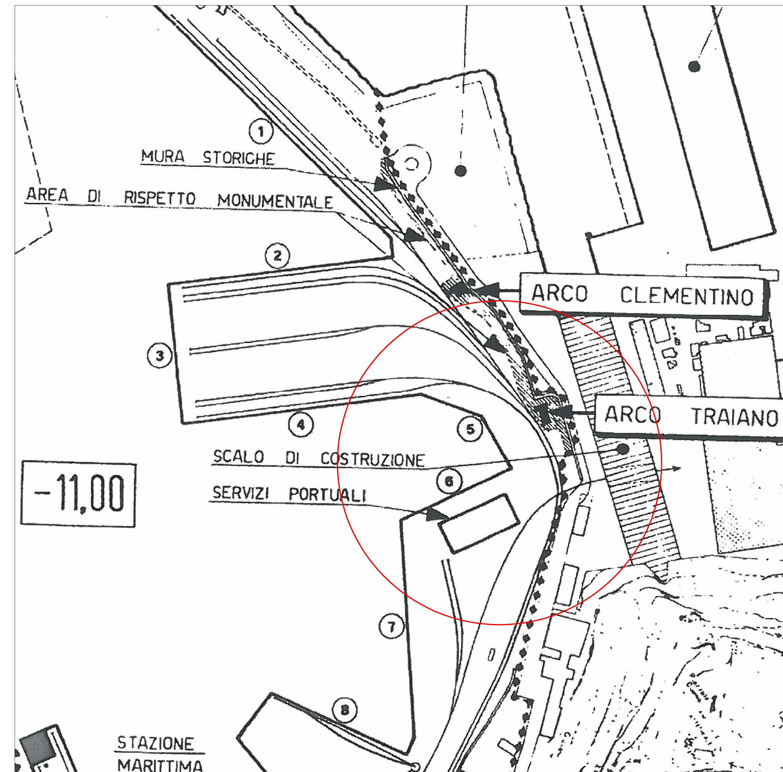
STRALCIO P.R.P. ATTUALE DELL'AREA DI INTERVENTO scala 1:2000
