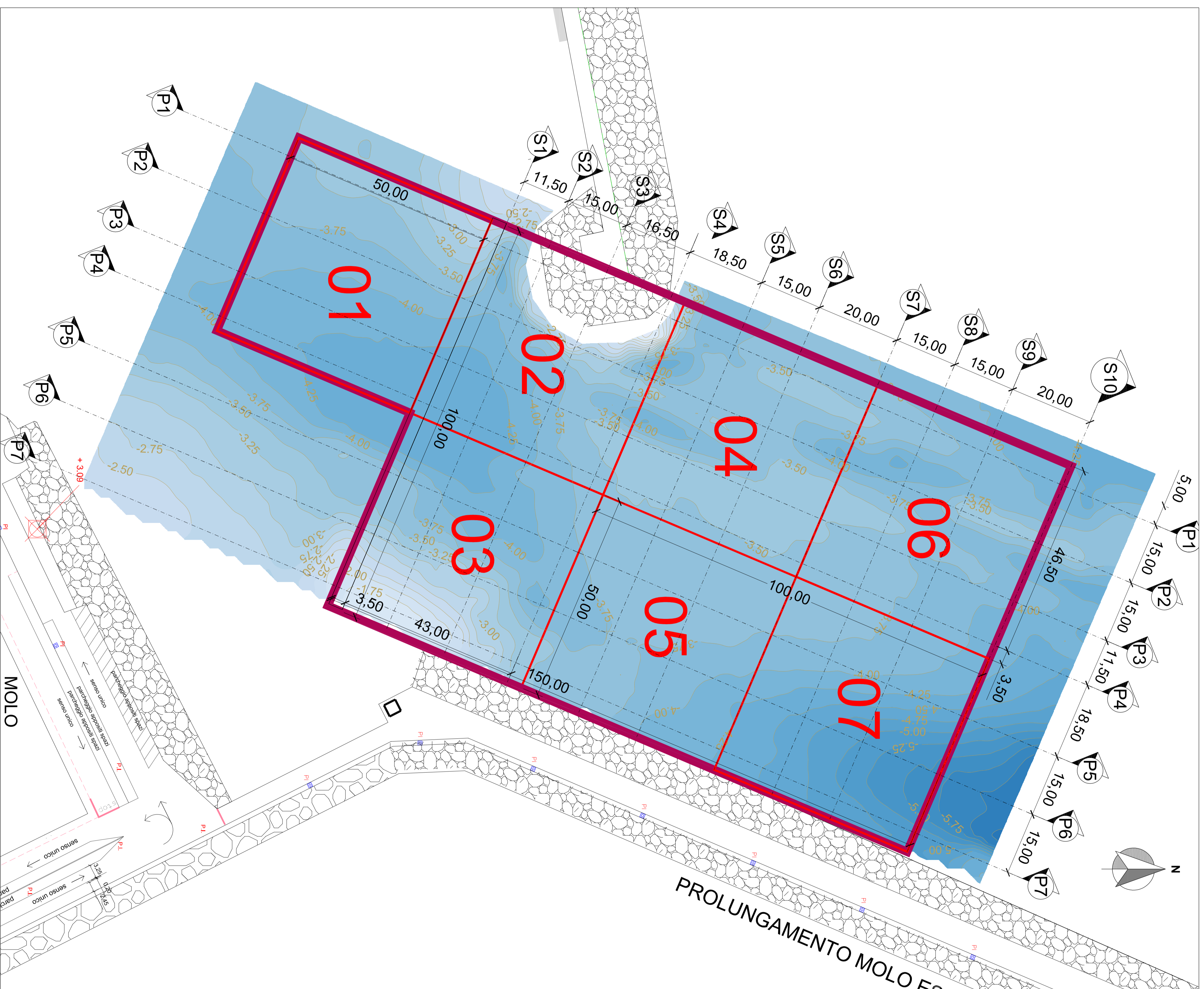
PLANIMETRIA CON BATIMETRIE scala 1:500
