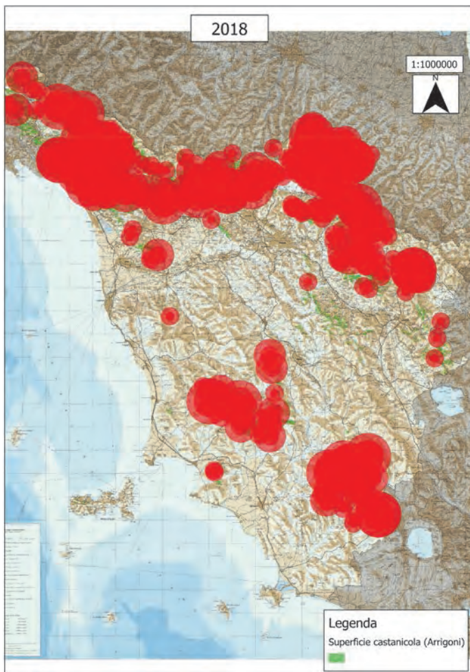
Simulazione diffusione sul territorio del Tormus sinensis 2018
